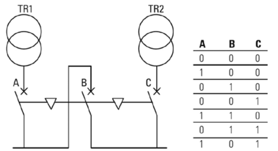
3'lü mekanik kilitleme (2 trafo 1 kuplaj)
