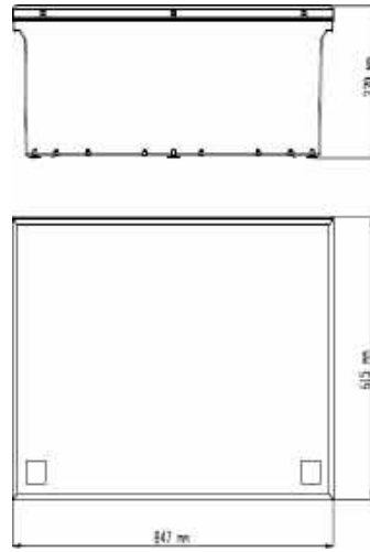
Dolapların İç Boyutları (mm)
